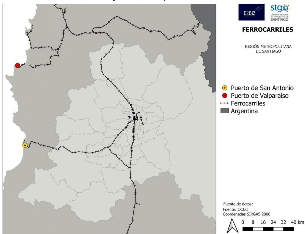
Figura N°57: Red ferroviaria
